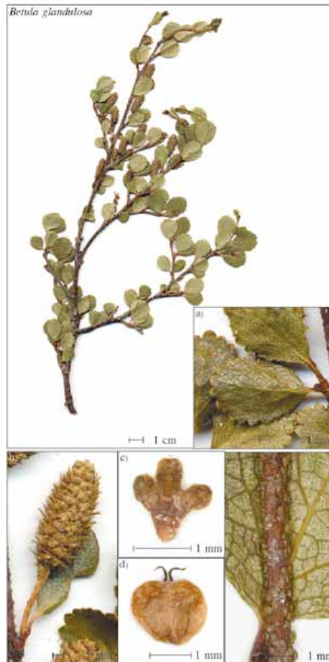
Betula glandulosa
